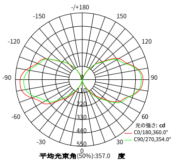
室内照明器具の配光曲線
