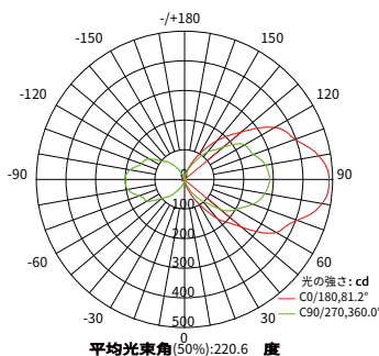
室内照明器具の配光曲線
